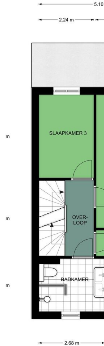
1e Verdieping, Gardameer 27 te Amersfoort De plattegronden zijn geschikt voor promotionele doeleinden. Er kunnen geen rechten aan ontleend worden. © Topr.n
