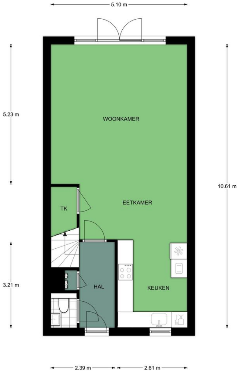
Begane grond, Gardameer 27 te Amersfoort De plattegronden zijn geschikt voor promotionele doeleinden. Er kunnen geen rechten aan ontleend worden. © Topr.n
