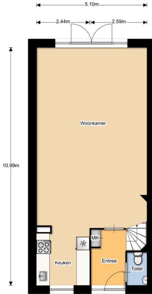
Begane grond
